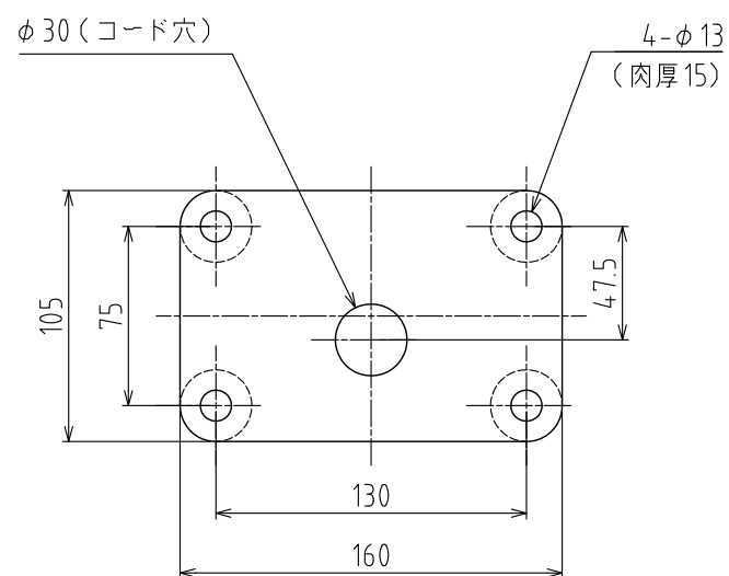
A矢視詳細 (S=1/2)
